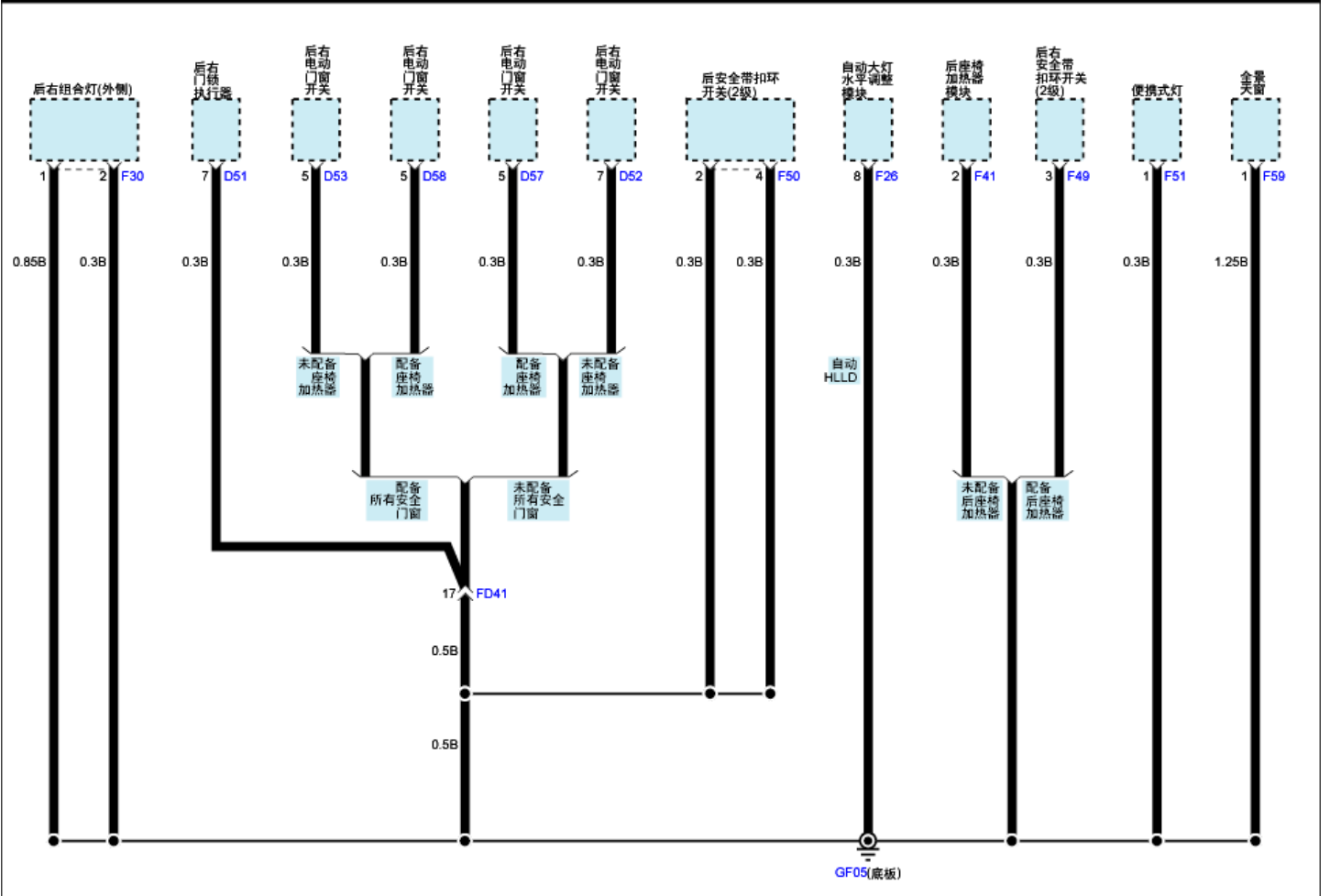
搭铁分布(13)
